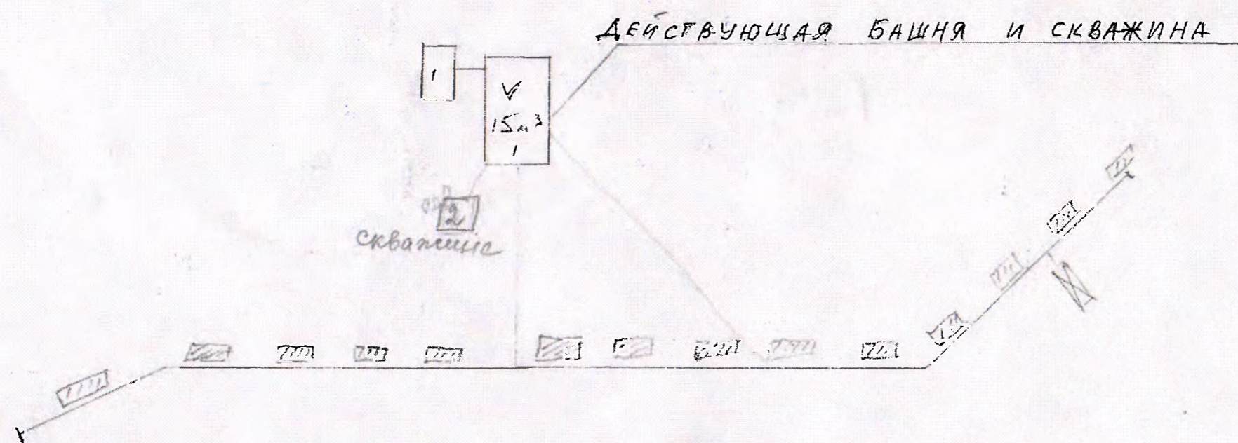
Схема водопровода х. Свиридов Медвенского района Курской области
